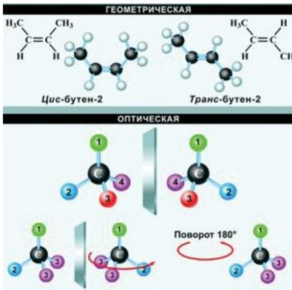
цис -1,2-дихлор- пропен
