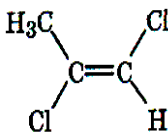
транс -1,2-дихлор- пропен
