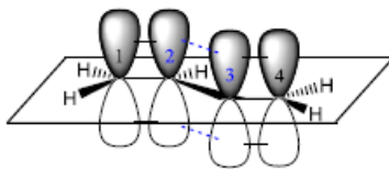
Рис.1. Схема образования \pi -связей в молекуле бутадиена-1,3
